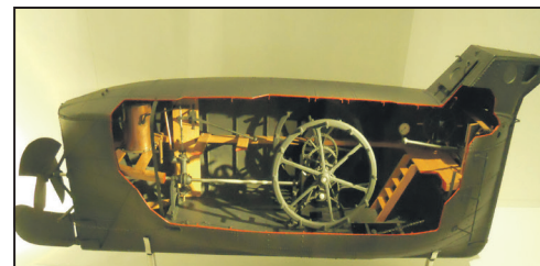
Modell des Brandtauchers. Quelle: https://de.wikipedia.org/wiki/Brandtaucher#/media/Datei:Brandtaucher,_Modell.jpg
