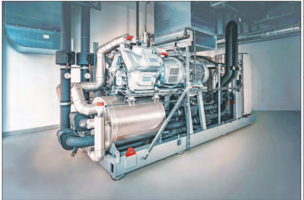
Die Energiezentrale ist das Prunkstück der Meerwasser-Wärmepumpe und Teil dieser umweltfreundlichen Technologie.
