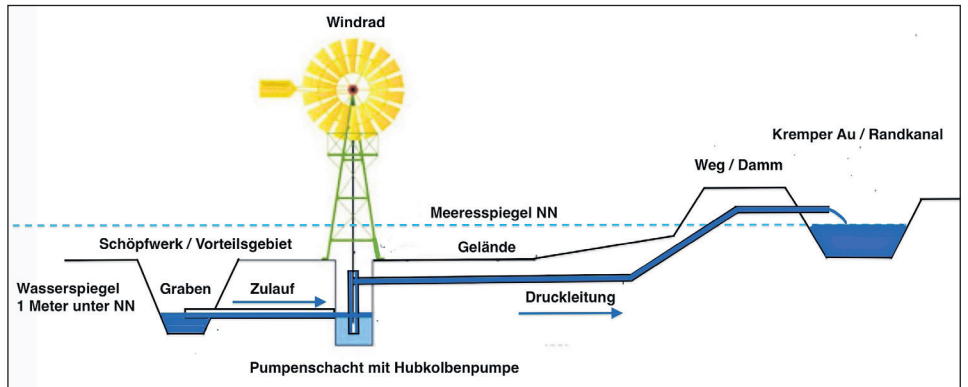
Funktionsweise der Windwasserpumpe. (Skizze: Wasser- und Bodenverband Neustädter Binnenwasser)
