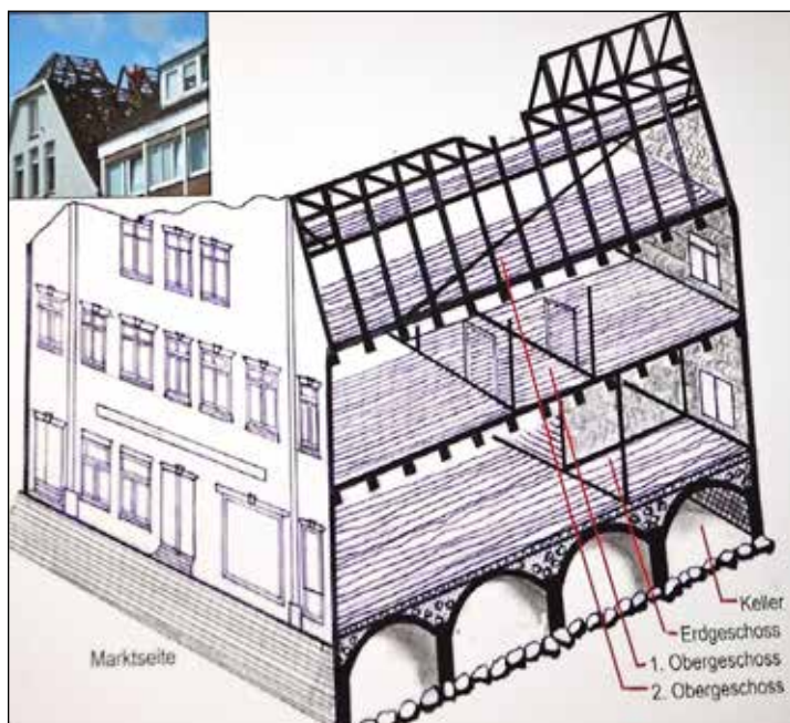
In einer idealisierten Darstellung von Klaus Schöllhorn ist das Haus als Längsschnitt zu sehen.
